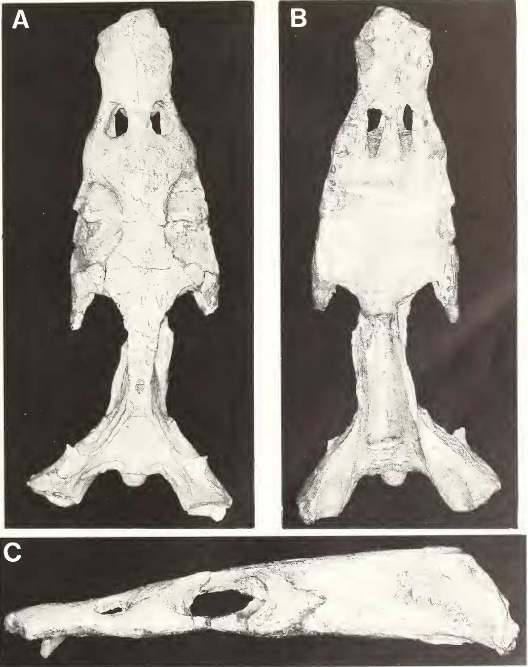
TEXT-FIG. 1. Nothosaurus juvenilis Edinger. Paläontologisches und Geologisches Institut und Museum, Universität Heidelberg, König Collection, K.8698-1 (holotype); Nusslocher Zementbruch, near Heidelberg; Lower Trochitenkalk (Anisian, Middle Triassic). A, dorsal view. B, ventral view. C, lateral view. All \times 1 .
